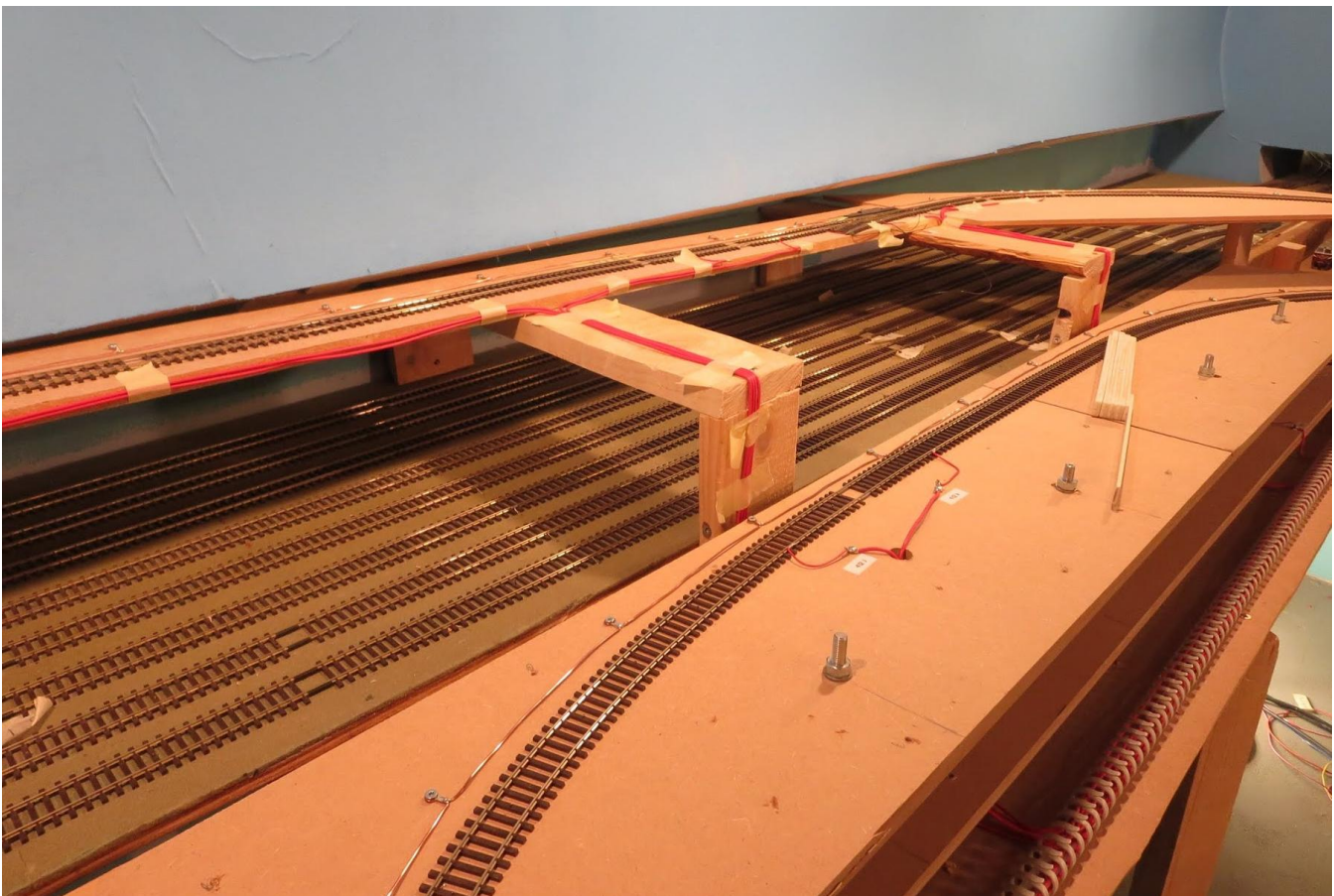
De røde kørestrømsledninger til forsyning af sporet, er trukket med en ledning til hvert spor. "o" lederen er et stykke uisoleret kobbertråd, lagt næsten ligesom tredjeskinen på spor o var det i gamle dage!
