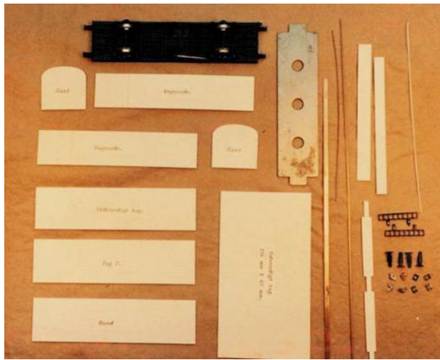
Alt, hvad der skal bruges for at bygge en Iks kølevogn. Th.: Vognens hoveddele er nu samlet, bemærk forlængelsen af undervognen.
