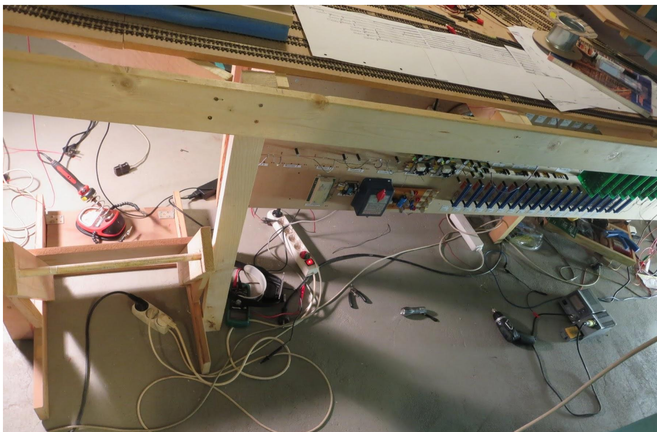
På den store tavle er de første printplader kommet på plads og som altid driller de i starten!
